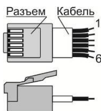
Вилка на кабель TP6P6C
