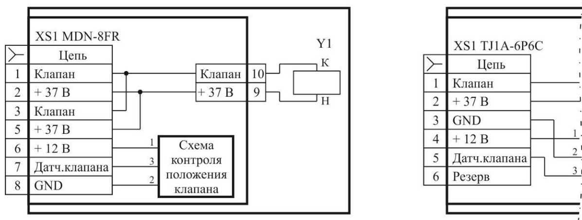
а) с разъемом MDN-8FR
