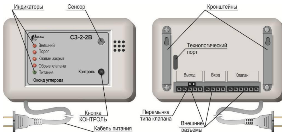
Рисунок 5 – Внешний вид сигнализатора типа СЗ-2-2В.
